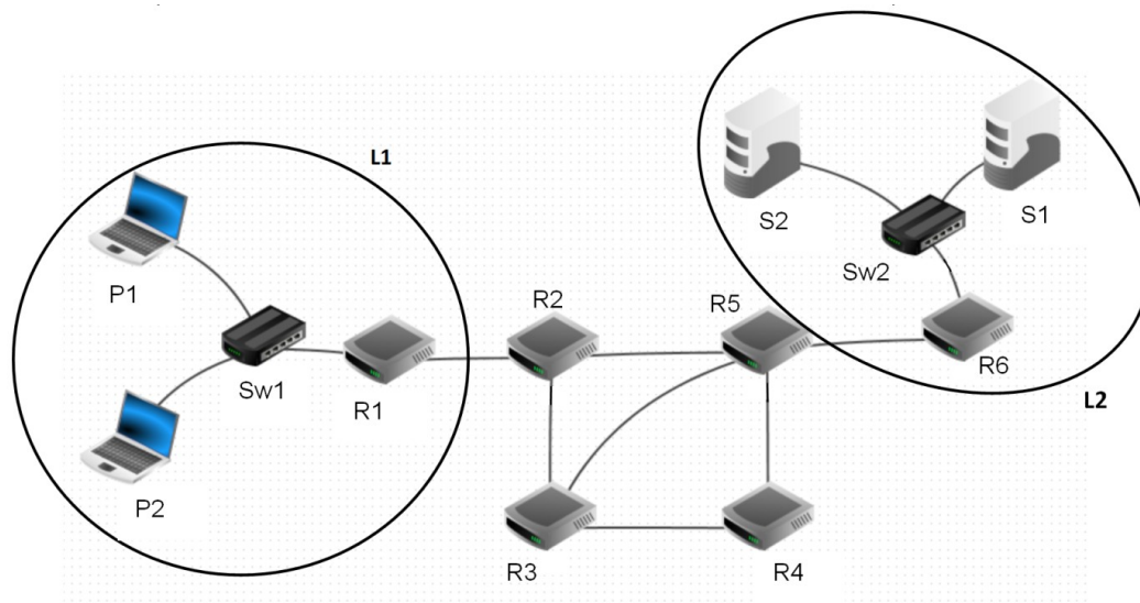
Figure 1 : Réseau d'entreprise
